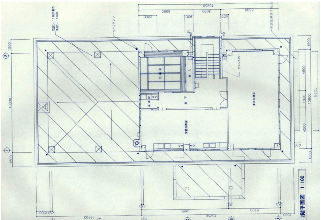
【川尻保健センター 2階図面（延床面積：約 161 m 2 ）】
